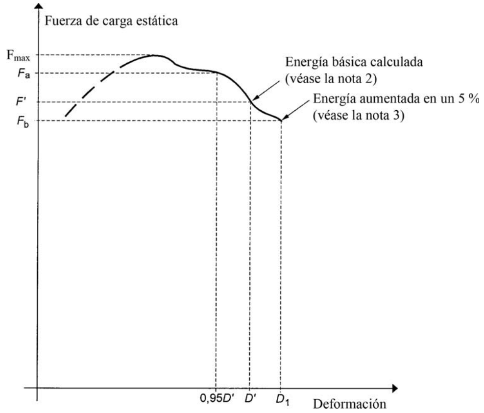
Figura 7.6 Curva de fuerza-deformación El ensayo de sobrecarga es necesario
