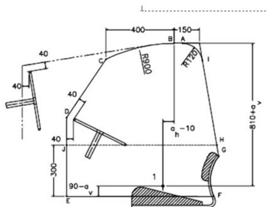
Figura 3.9.a Vista lateral sección en el plano de referencia
