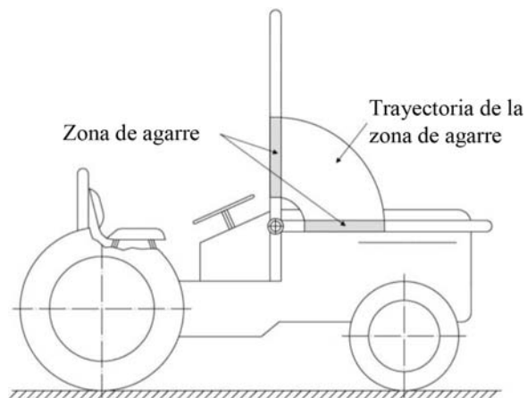
Figura 6.20 Zona de agarre
