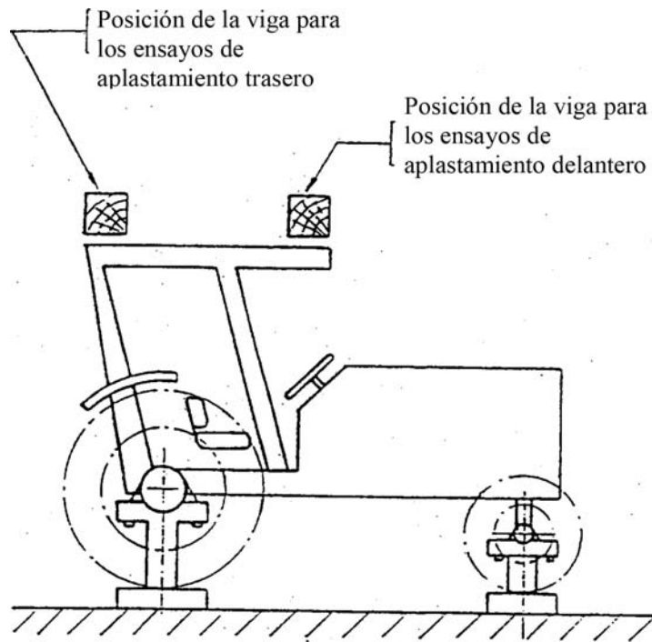
Figura 4.7.d Cabina de protección
