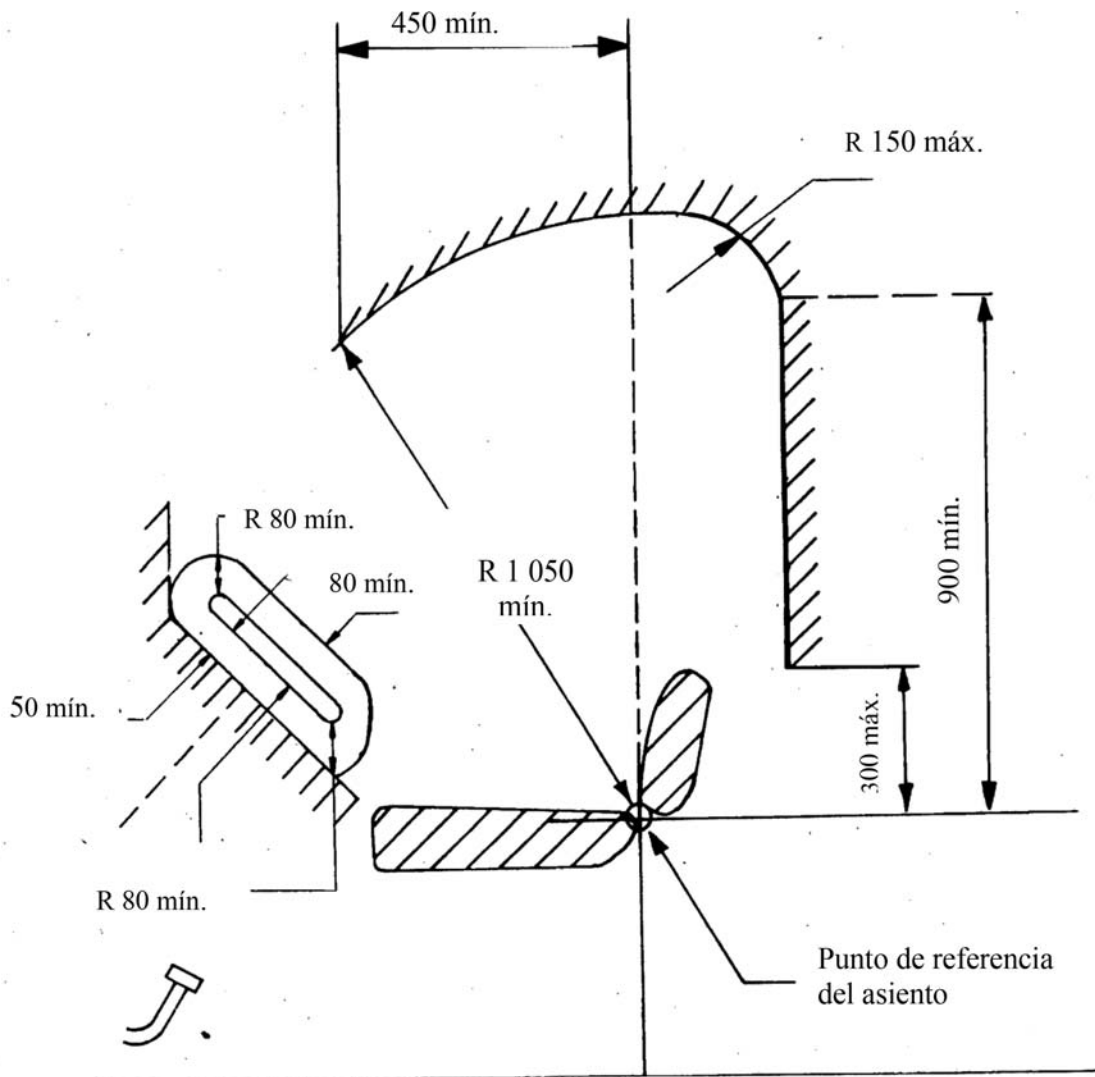
Figura 2 (Dimensiones en milímetros)
