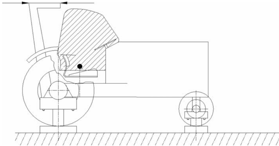
Marco de barras antivuelco trasero
