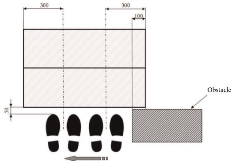
Figura 7.11 Envoltura de las zonas accesibles (Dimensiones en mm)
