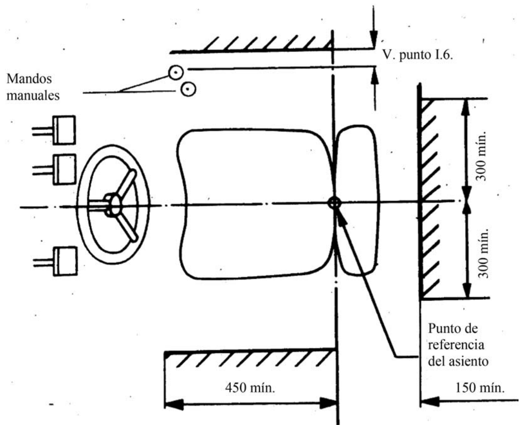
Figura 3 (Dimensiones en milímetros)
